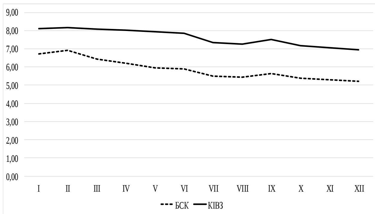
Рис. 1. Сезонна динаміка середньорічних показників БСК (мг/дм³) та КІВЗ
