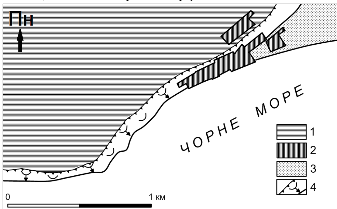
Рис. 3. Західний фланг Тилігульського пересипу: 1 – суша, 2 – "курені", 3 – тіло пересипу, 4 – активні абразійно-зсувні кліфи.
